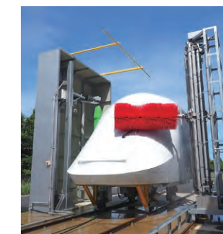
電車用先頭洗浄装置 (製作依頼元：株式会社アサヤマ)
